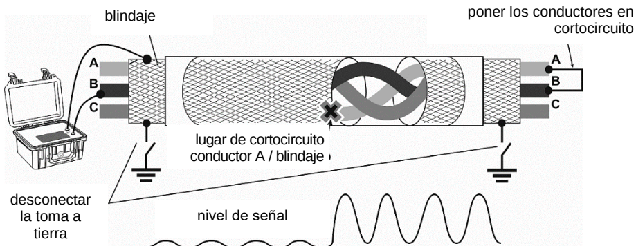
Fig. 37. Esquema de conexión del transmisor y la detección del lugar entre el conductor y el blindaje del cable
