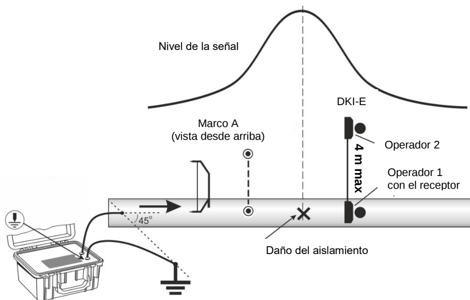
Fig. 35. Esquema de conexiones y fuerza de la señal durante la localización del daño en el aislamiento a través del aumento de la señal
