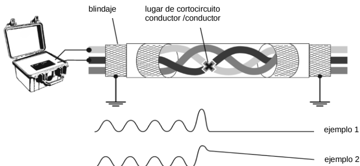
Fig. 36. Esquema de conexión del transmisor y la detección del lugar entre los conductores
