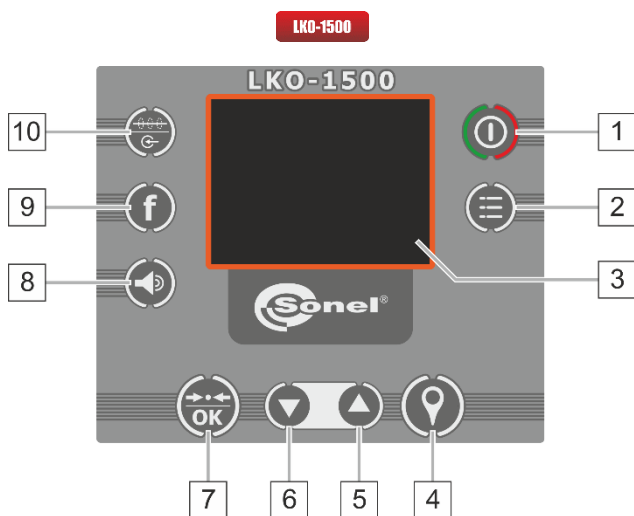
Fig. 10. Panel del receptor LKO-1500
