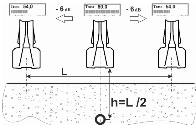
Fig. 30. Medición de profundidad con el método indirecto "-6dB" (LKQ-1500)
