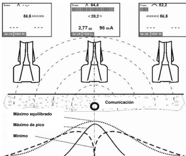
Fig. 23. Cambio de nivel de la señal con el desplazamiento del receptor hacia un lado del trazado de la línea
