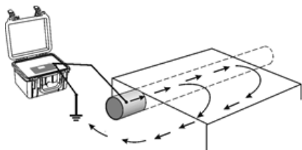
Fig. 3. Conexión del transmisor a la tubería
