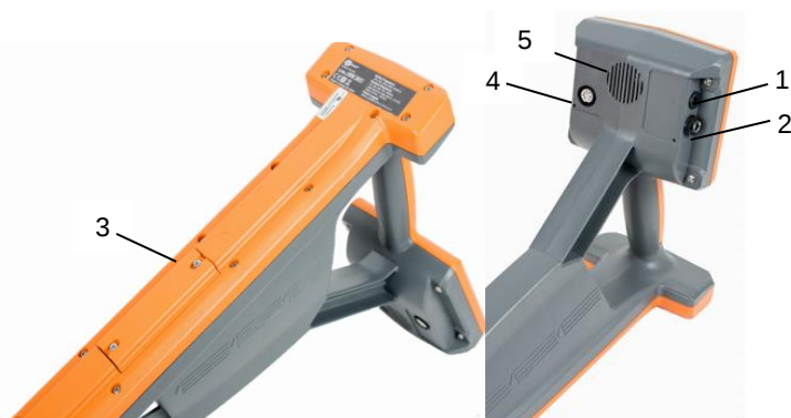
Fig. 7. Aspecto y marcaje de tomas del receptor
