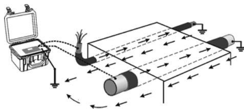
Fig. 4. Conexión del transmisor al blindaje del cable con la toma a tierra o a la tubería
