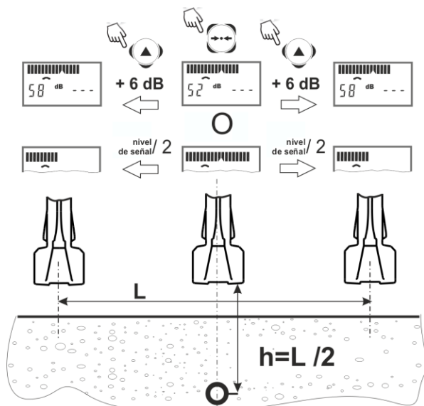
Fig. 29. Medición de profundidad con el método indirecto "-6dB" (LKQ-1500-LITE)
