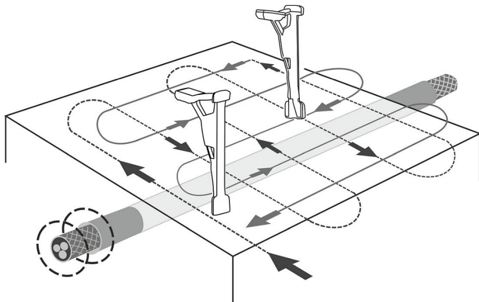
Fig. 31. Estudio del terreno sin el uso del transmisor LKN
