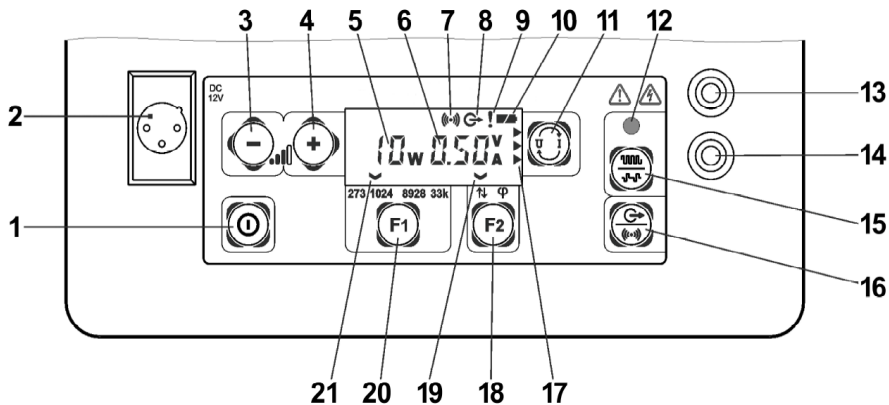
Fig. 2. Panel frontal del transmisor LKN-1500
