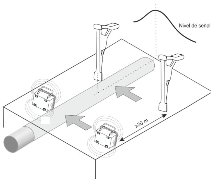
Fig. 33. Estudio del terreno con el uso de LKN-1500
