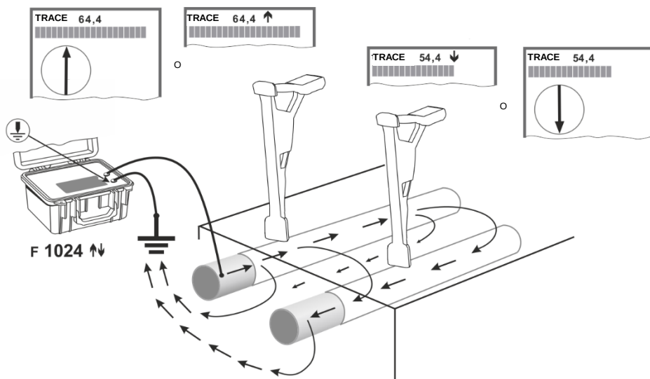
Fig. 26. Dirección de la corriente y lecturas del localizador en las tuberías separadas galvánicamente
