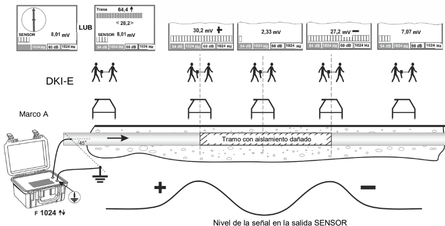
Fig. 34. Esquema de conexiones y fuerza de la señal durante la localización del daño en el aislamiento a través de la detección de la caída de la señal con el cambio del signo de polaridad
