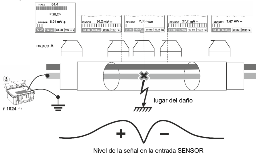
Fig. 38. Esquema de conexión del transmisor y la detección del lugar entre el conductor y el blindaje del cable
