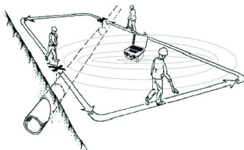
Fig. 32. Estudio del área utilizando el transmisor en modo inductivo
