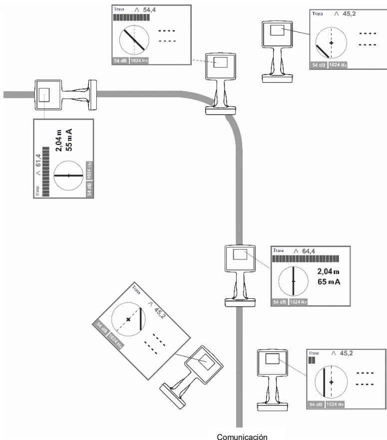
Fig. 25. Búsqueda con la opción "Brújula, línea"
