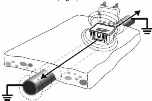
Fig. 5. Excitación inductiva de la corriente en el objeto examinado
