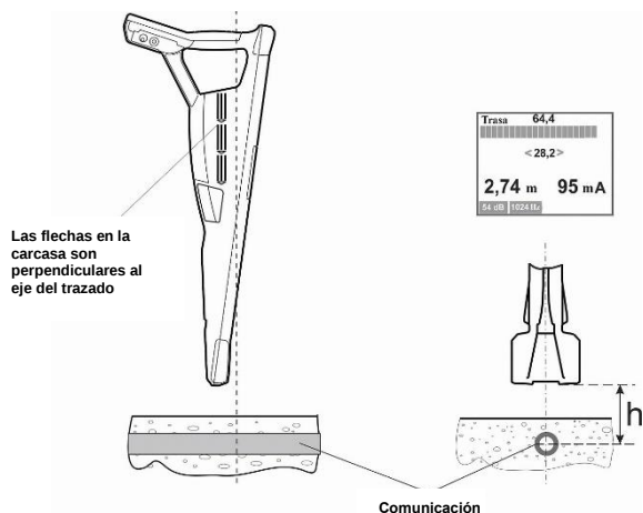
Fig. 28. Medición directa de la profundidad
