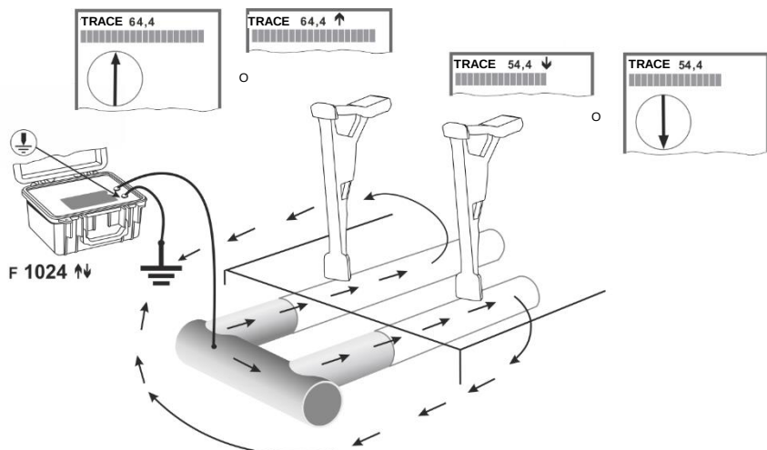
Fig. 27. Dirección de flujo de la corriente en los tubos conectados galvánicamente
