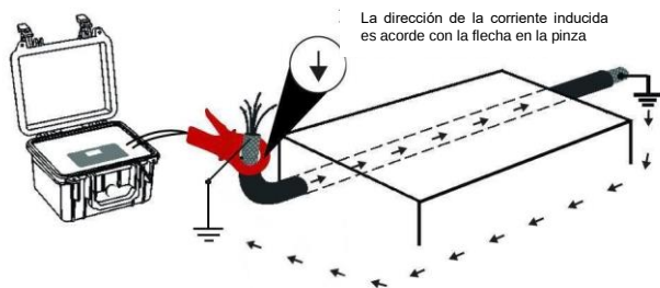
Fig. 6. Excitación inductiva de la corriente en el objeto examinado con el uso de las pinzas de transmisión
