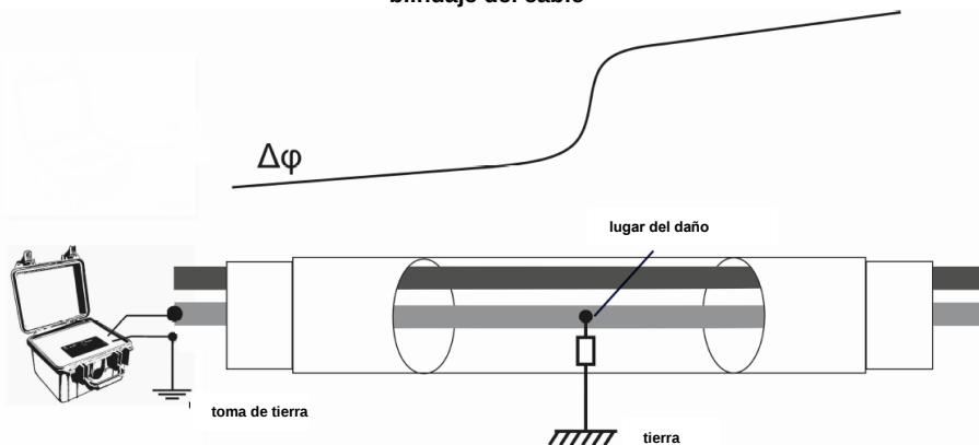
Fig. 38. Esquema de conexión del transmisor y la detección del lugar entre el conductor y el blindaje del cable
